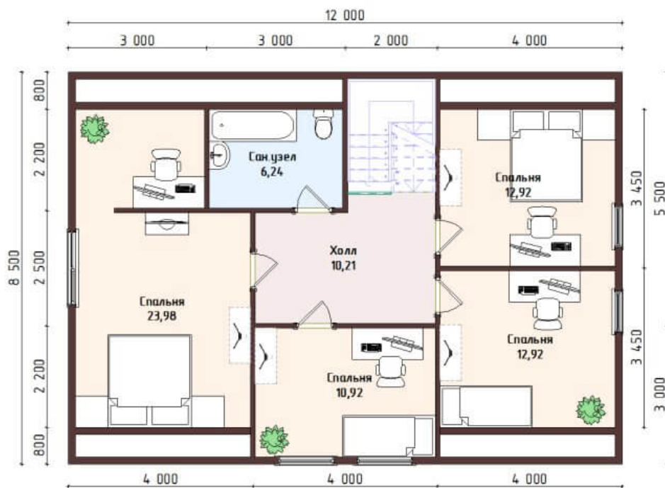
План 2-ого этажа
