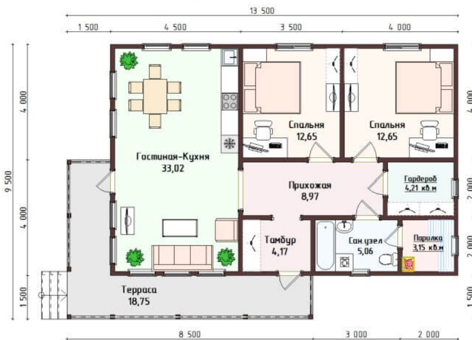
План 1-ого этажа
