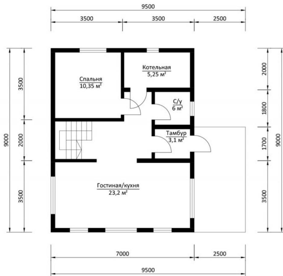
План 1 этажа
