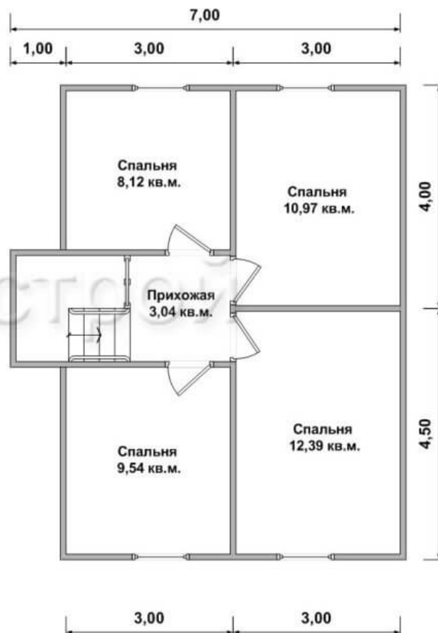
План 2-ого этажа
