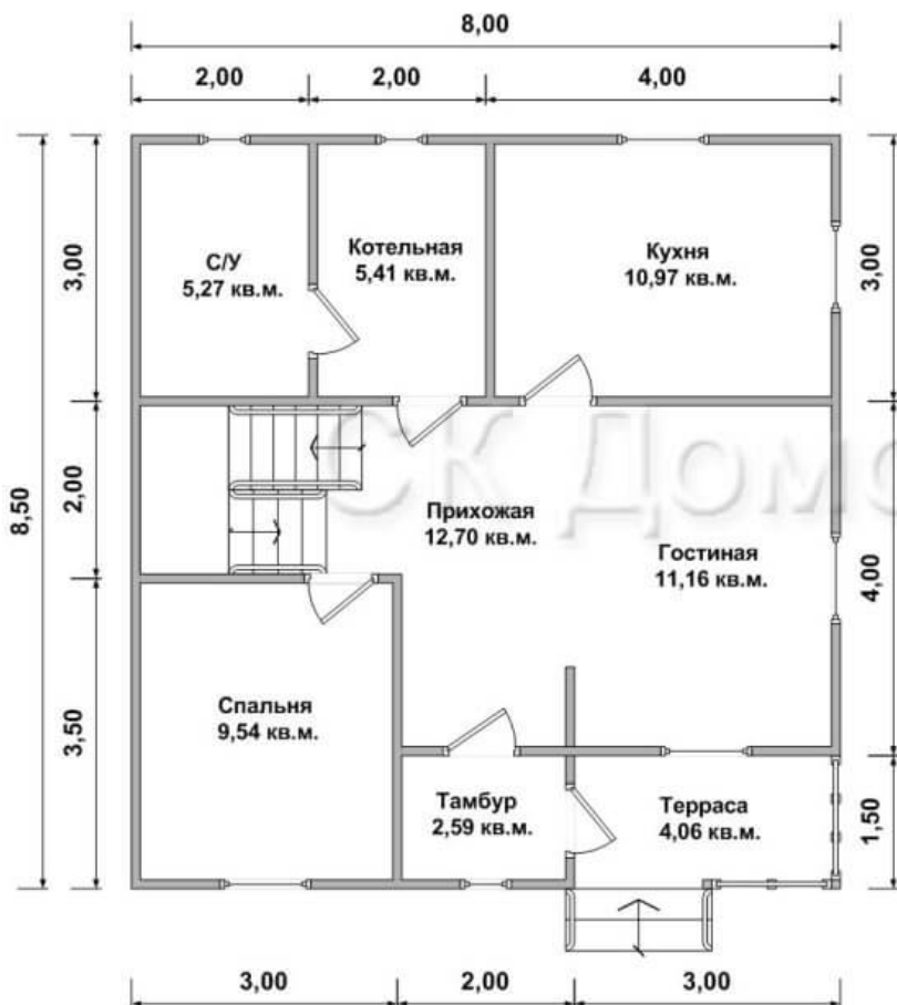
План 1-ого этажа
