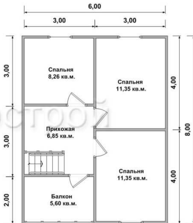
План 2-ого этажа
