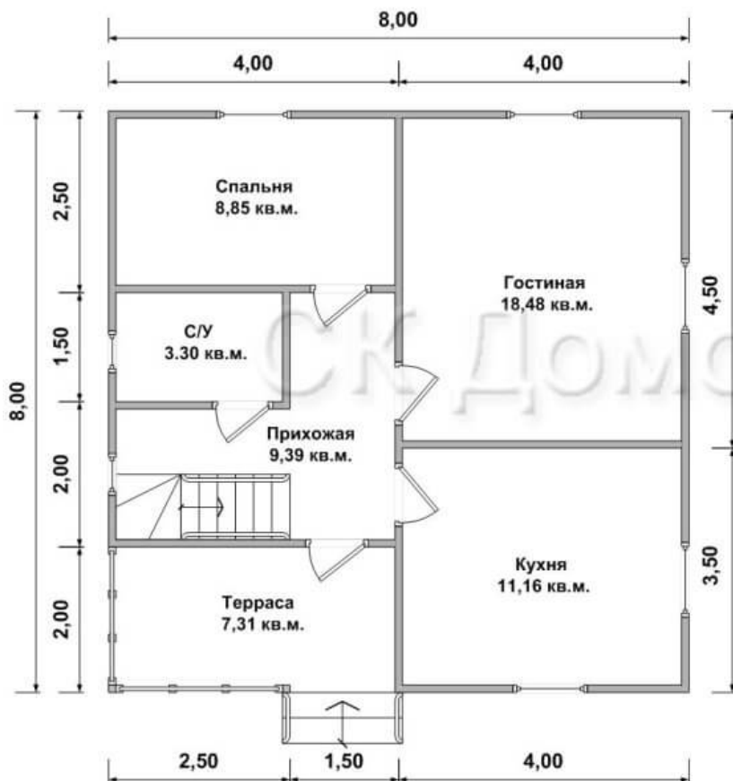
План 1-ого этажа
