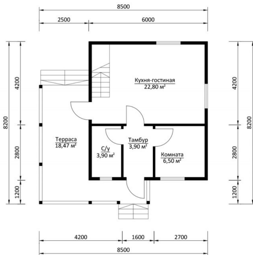
План 1 этажа
