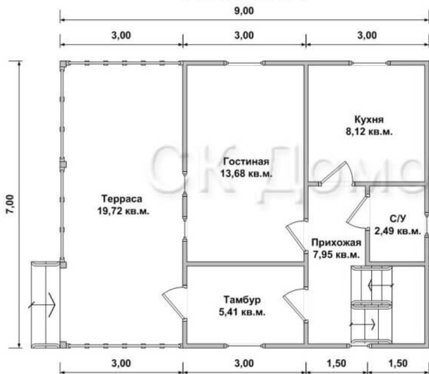
План 1-й этаж
