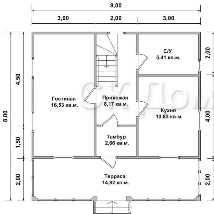
1-й этаж
