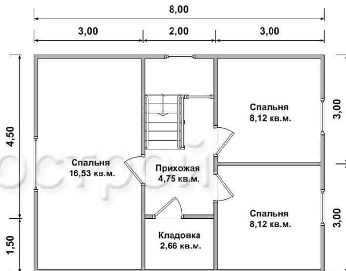
2-й этаж
