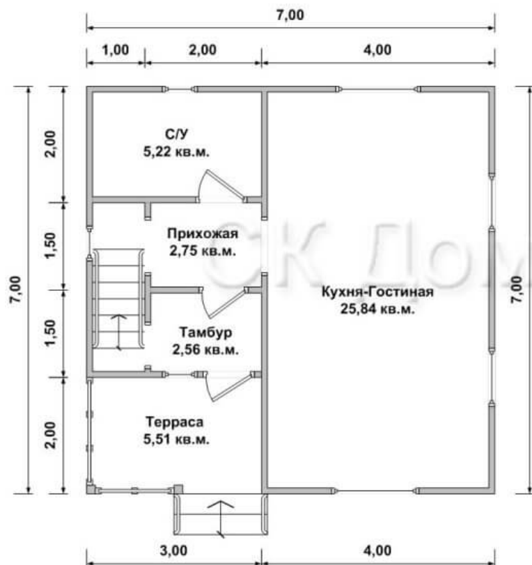
План 1-й этаж
