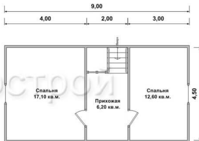
План 2-ого этажа
