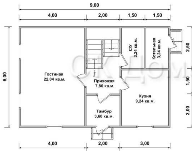
План 1-ого этажа
