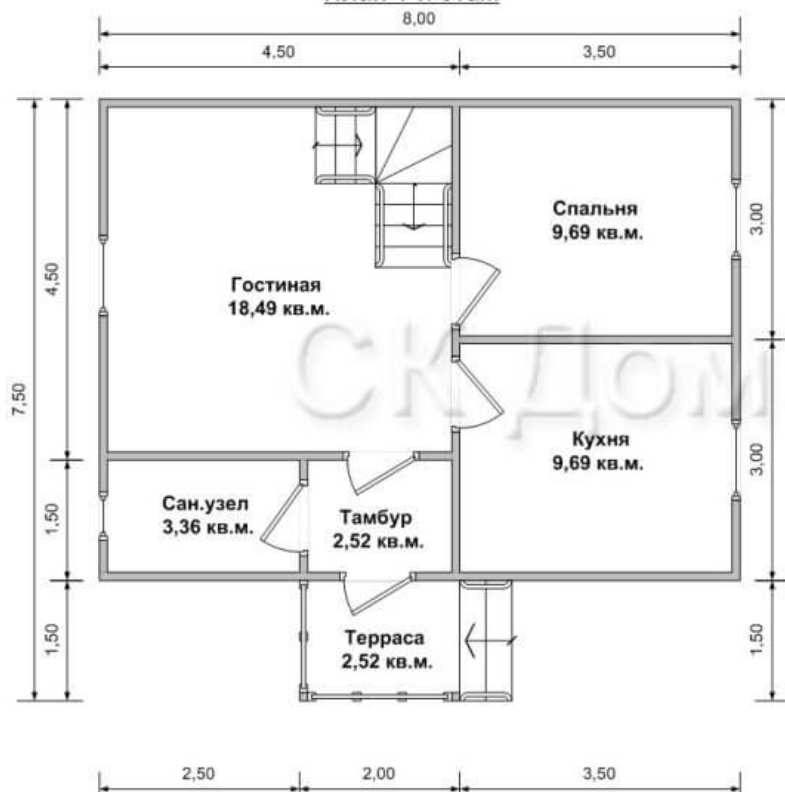
План 1-й этаж
