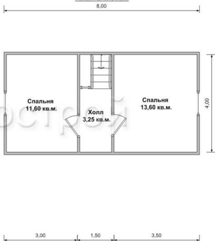
План 2-й этаж
