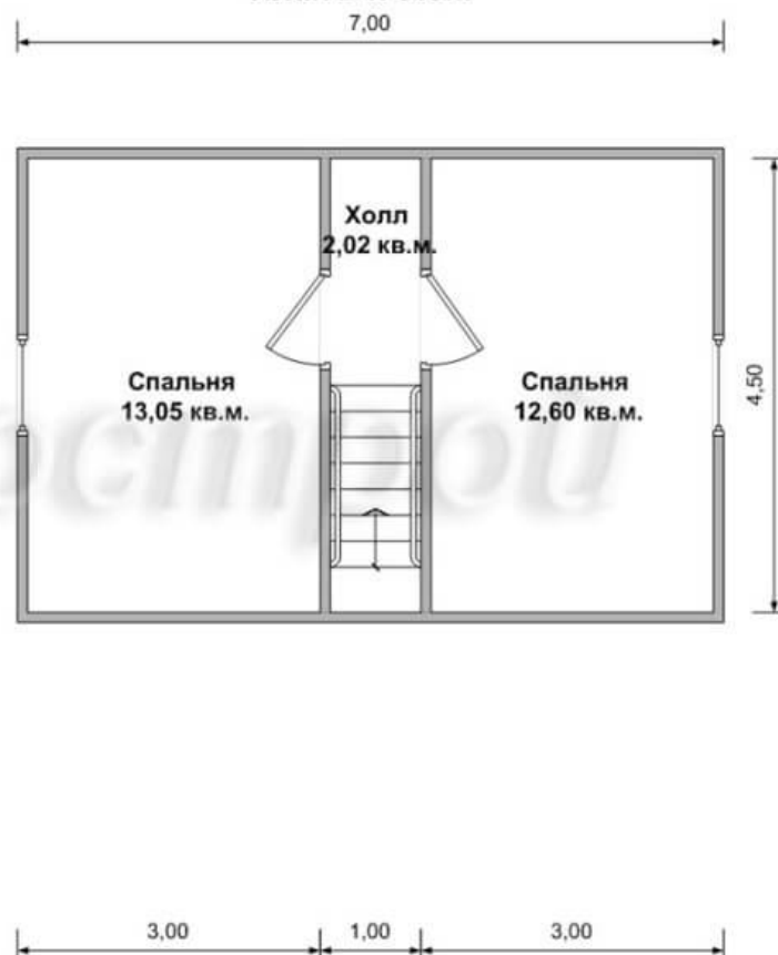
План 2-й этаж
