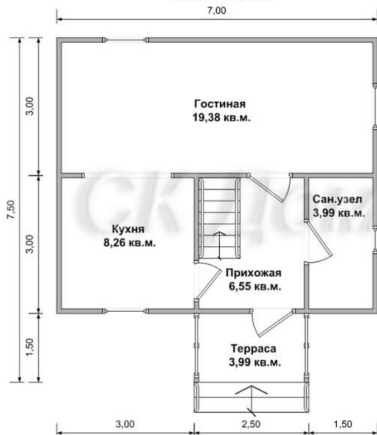
План 1-й этаж
