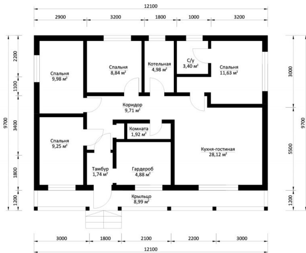
План 1 этажа
